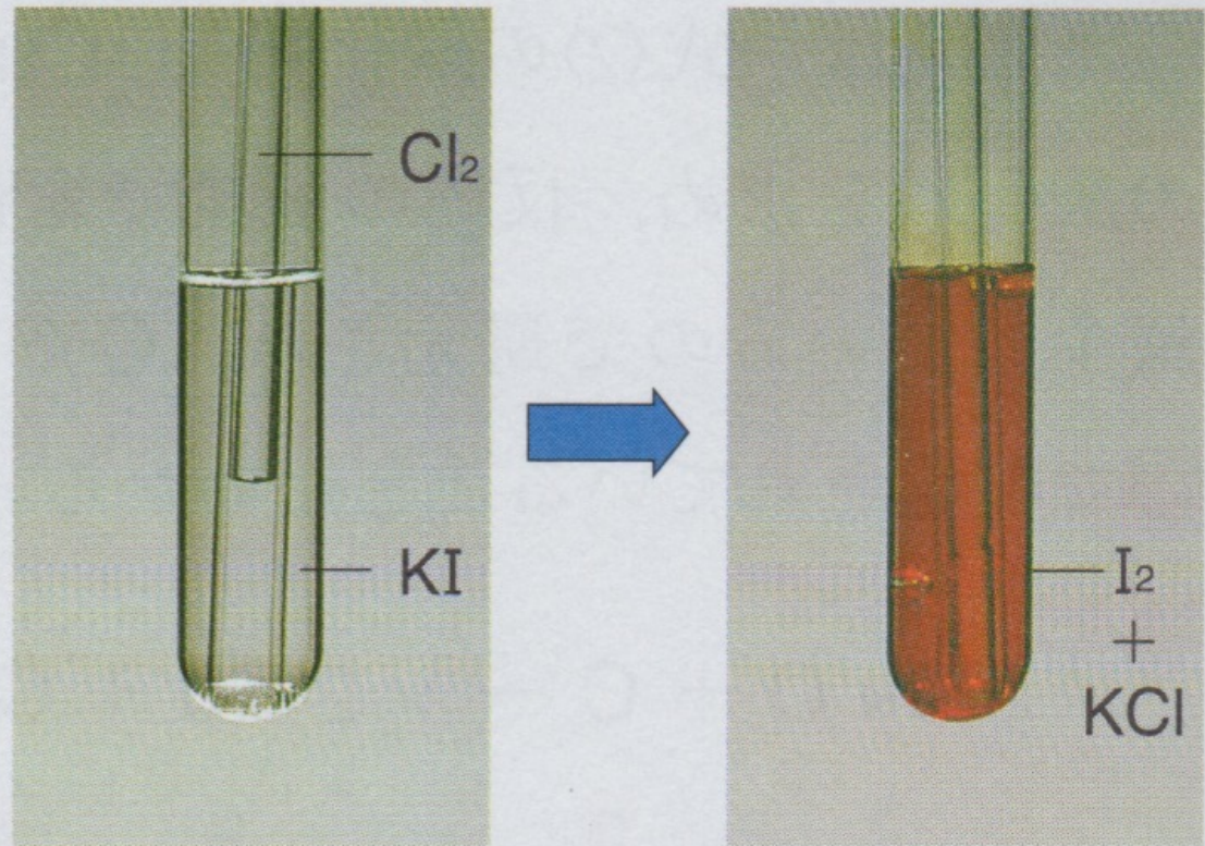
図5 ヨウ化カリウム水溶液と塩素 の反応 褐色はヨウ素 (I 2 ) の色
