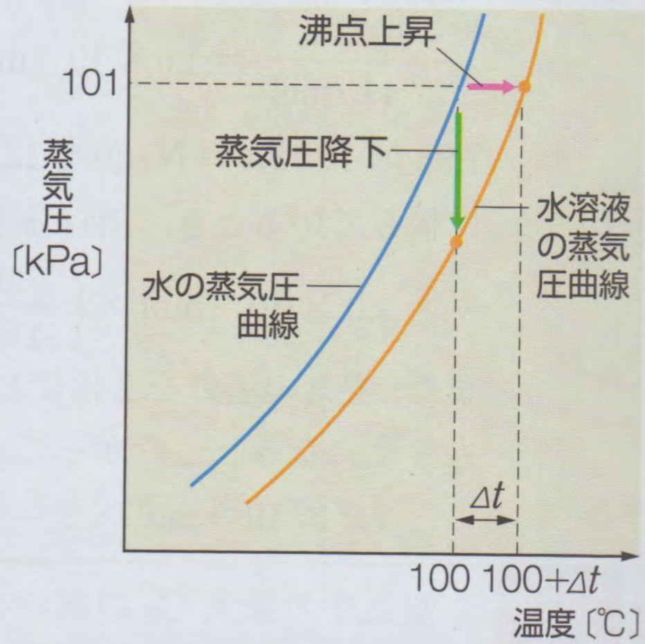
図13 蒸気圧降下と沸点上昇
