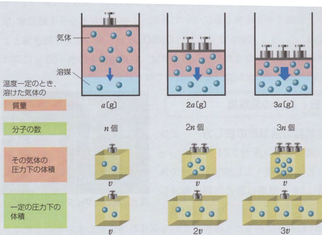
図11 ヘンリーの法則
