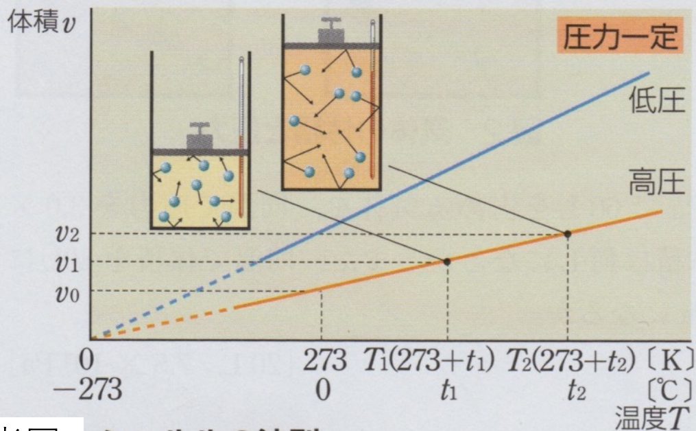
参考図 シャルルの法則
